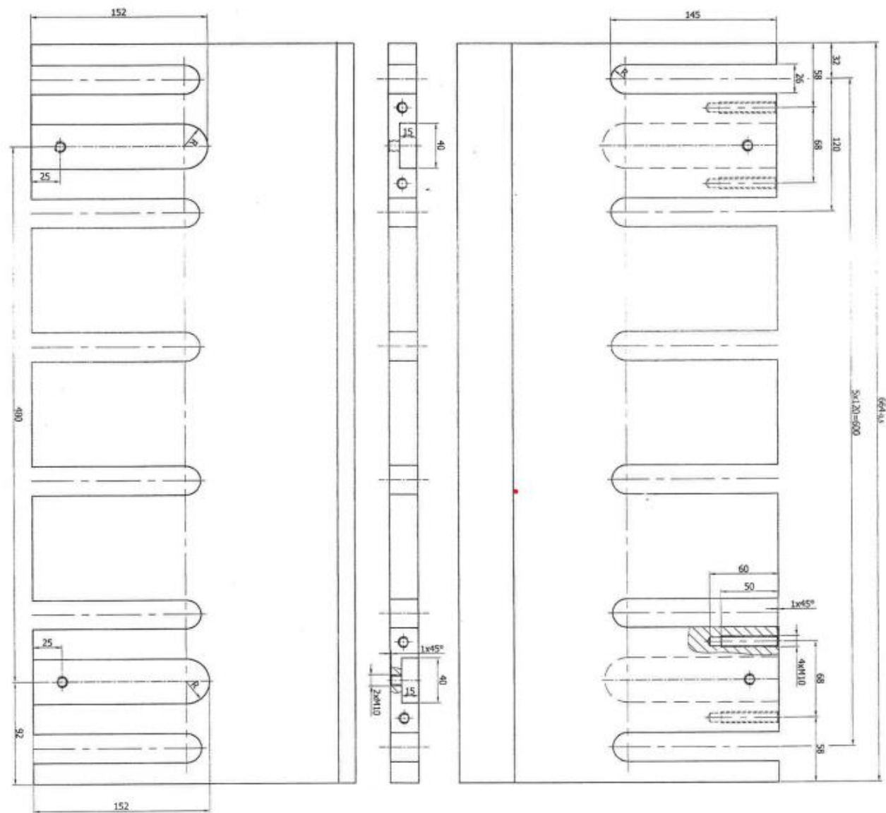
Rysunek noża tnącego:
